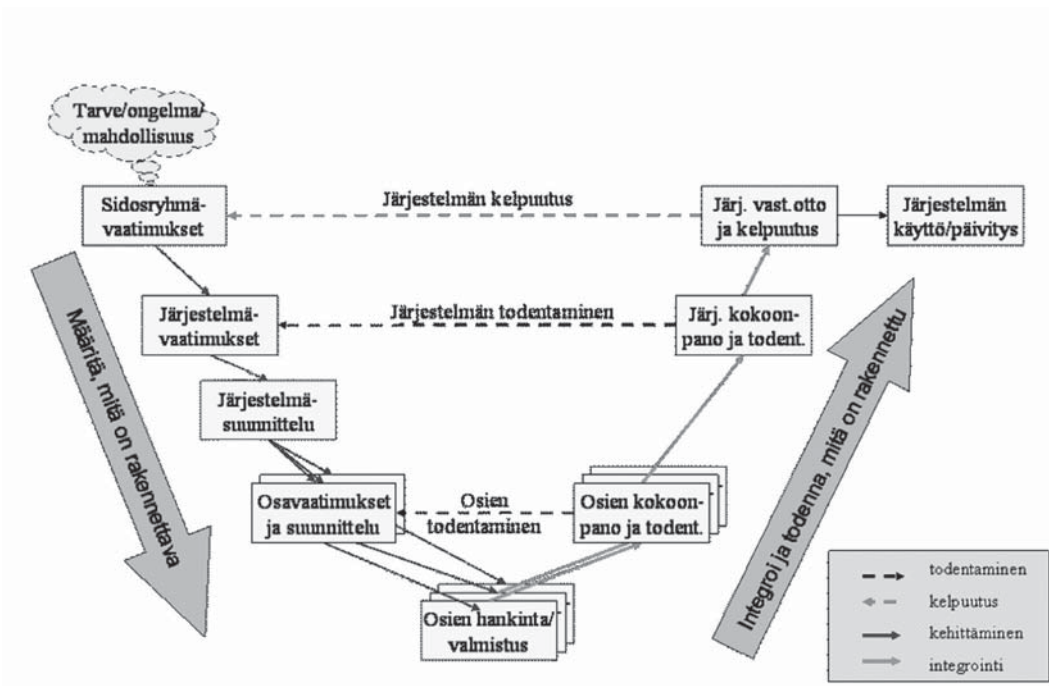
Kuva 1-1. Järjestelmätekniiikan V-malli.
