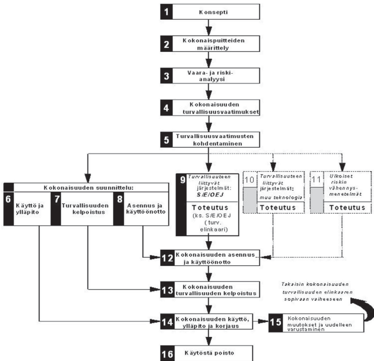
Kuva 24. Elinkaarimallin vaiheet (IEC 61508-1).
