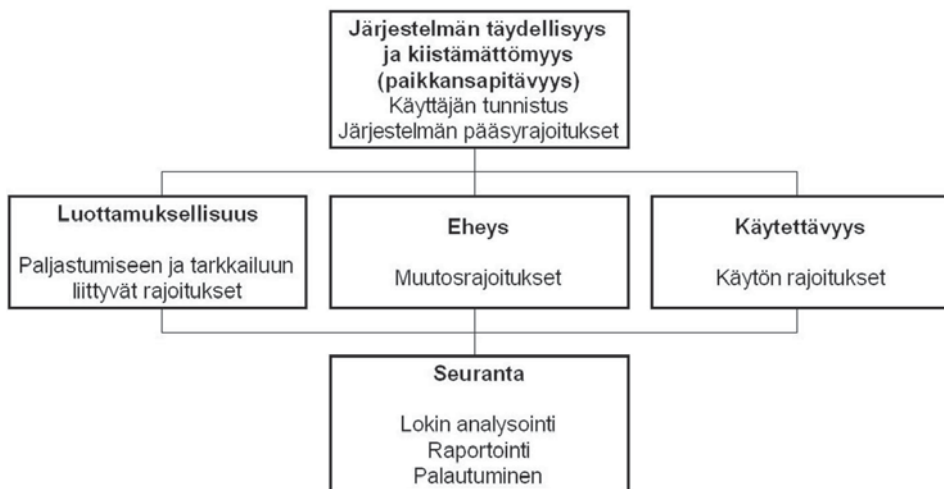
Kuva 5. Tietoturvan tavoitteet.
