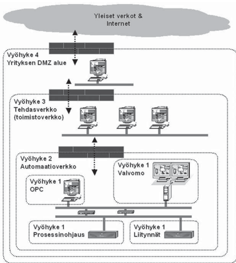
Kuva 25: Syvyysuuntainen suojaus.
