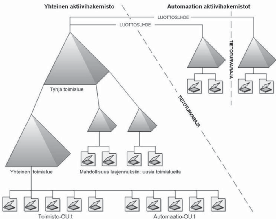
Kuva 3-1. Aktiivihakemiston rakenne.
