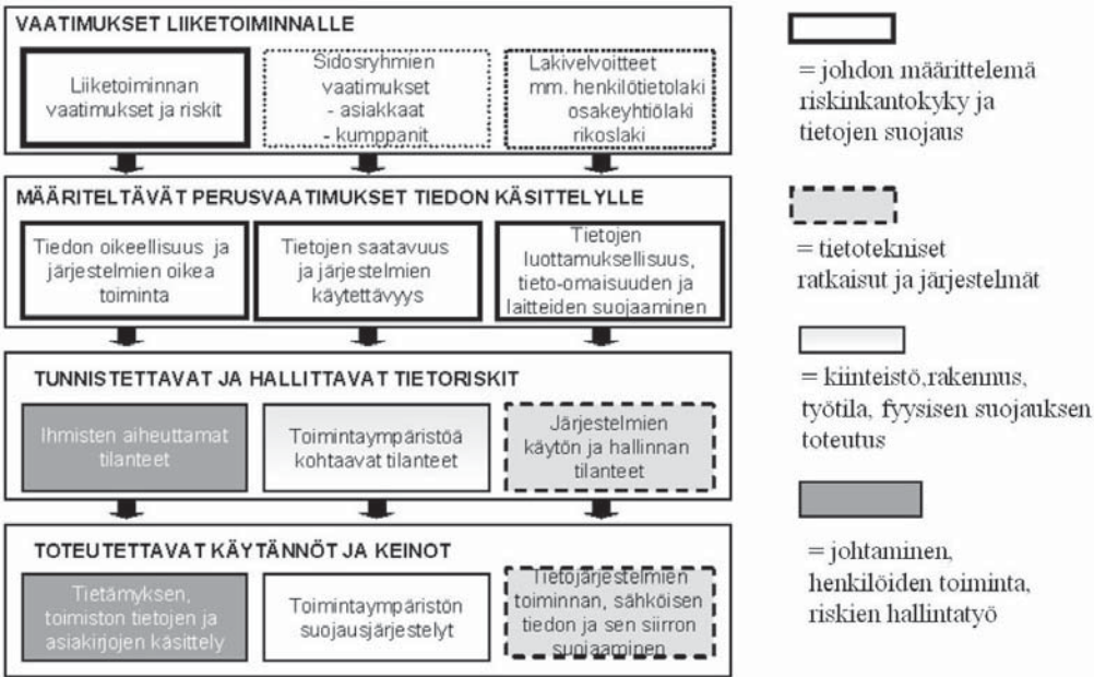
Kuva 8. Tietoturvavaatimusten määrittely.
