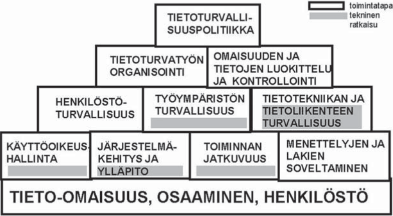
Kuva 7. Tietoturvan hallintajärjestelmä.
