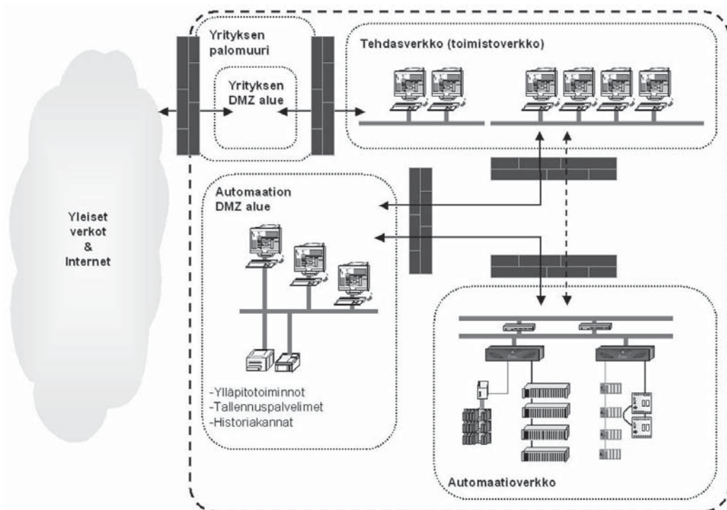
Kuva 28. Ei-kenenkään-maa-malli.
